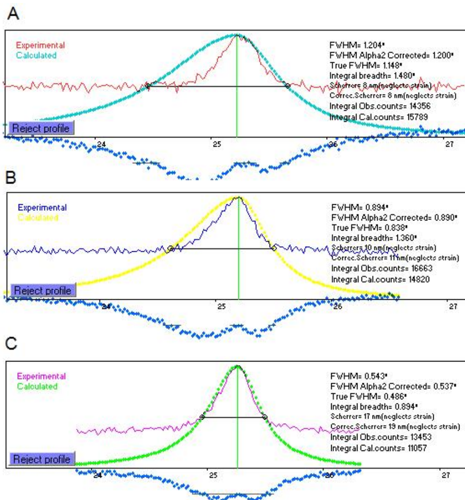
Gambar 3. Hasil perhitungan ukuran kristalit TiO 2 berdasarkan persamaan Scherer menggunakan software Xpowder
