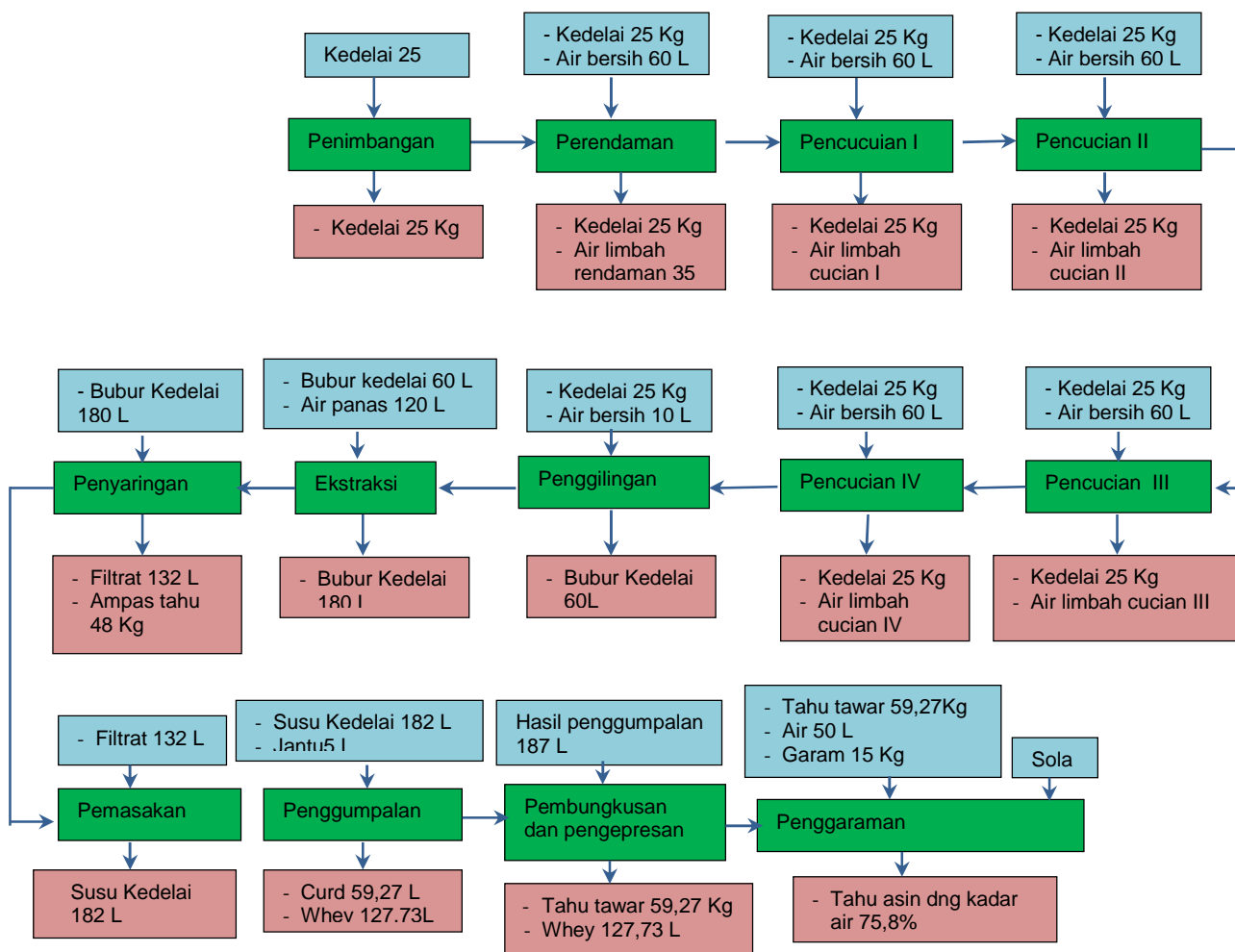
Gambar 1. Neraca Massa Proses Pembuatan Tahu
